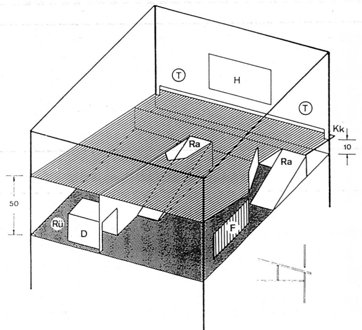
Abb. 1: Mastgruppenhaltungsanlage
