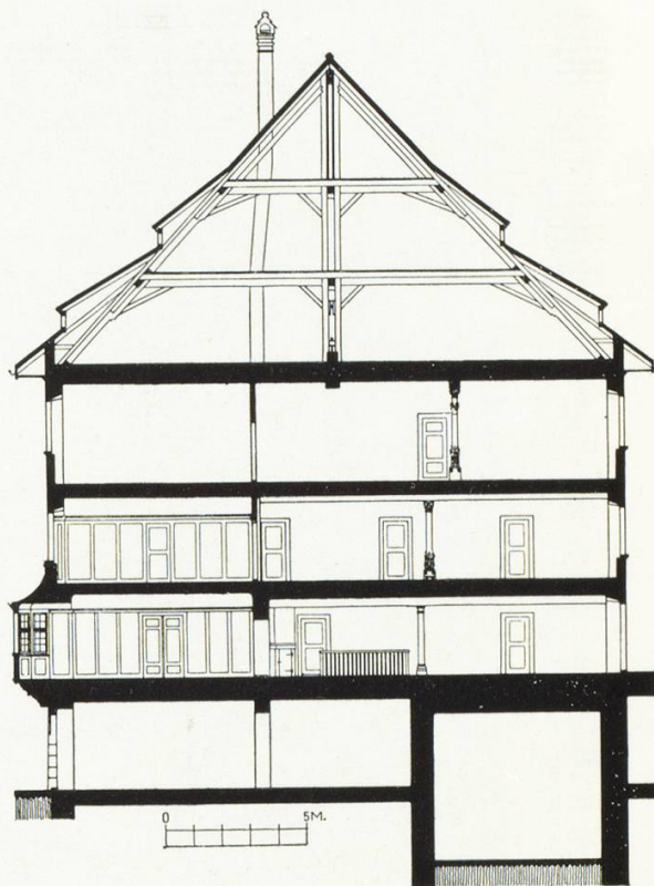
Schnitt
