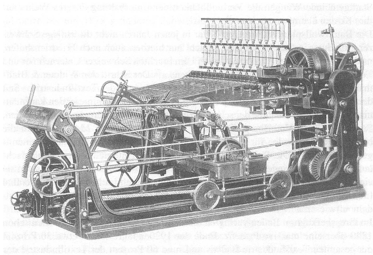
Die Baumwollspinnerei Wangen arbeitete mit Maschinen der Firma Rieter, die finanziell an der Spinnerei beteiligt war. Im Bild ein Rieter-Selfactor von 1860, also aus der Zeit, als das Unternehmen in Wangen gegründet wurde. (Bild Historisches Archiv der Maschinenfabrik Rieter AG)
