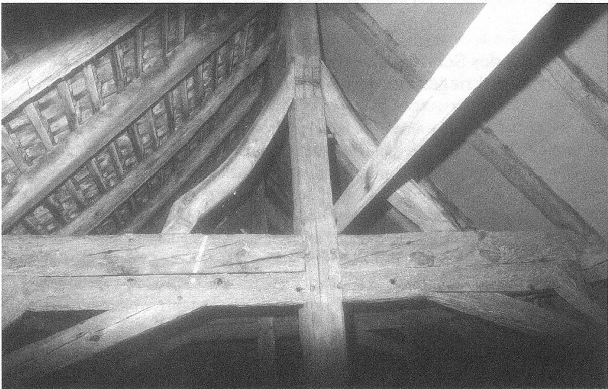
Abb. 11: Blick in den letztmals 1690 umgebauten Dachstuhl des Kirchenschiffes. Damals wurden Föhrenhölzer anstelle älterer Eichenhölzer eingesetzt. Von 1515 stammen unter anderem die Hängesäulen mit den charakteristischen, verdickten Knotenpunkten. Noch älter sind wiederverwendete Hölzer von 1306, 1412 und 1421.
