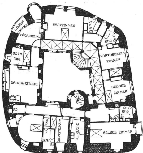
Grundriss vom ersten Obergeschoß
