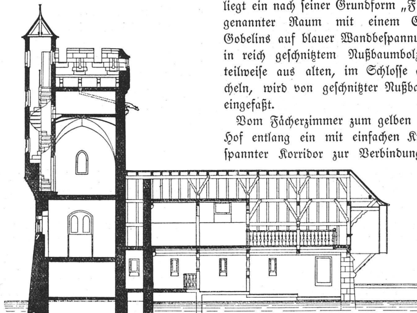
Längsschnitt. — Maßstab 1 : 200
