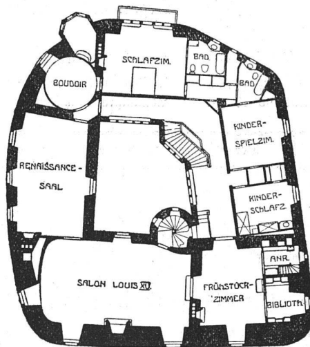
Grundriss vom zweiten Obergeschoß
