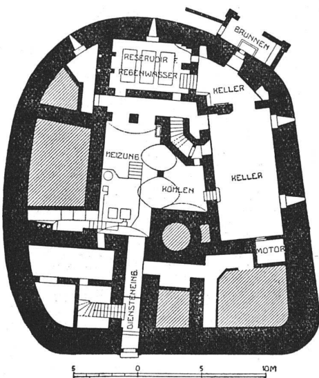
Grundriss vom Keller
