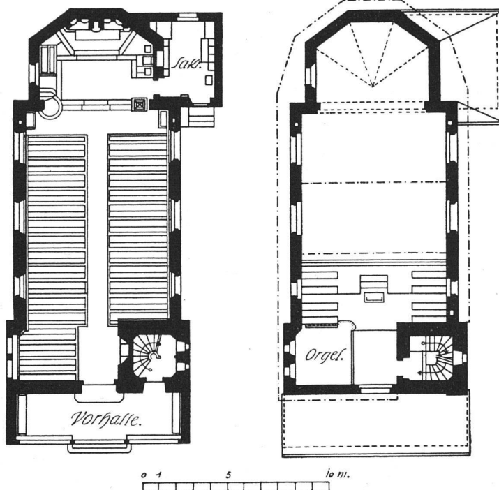
Die katholische Kirche in Trimbach. — Grundrisse vom Erdgeschoß und der Empore. — Maßstab 1:300
