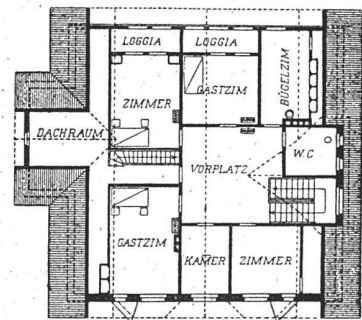
Das Haus Nind in Winterthur. — Grundrisse. — Maßstab 1:400.
