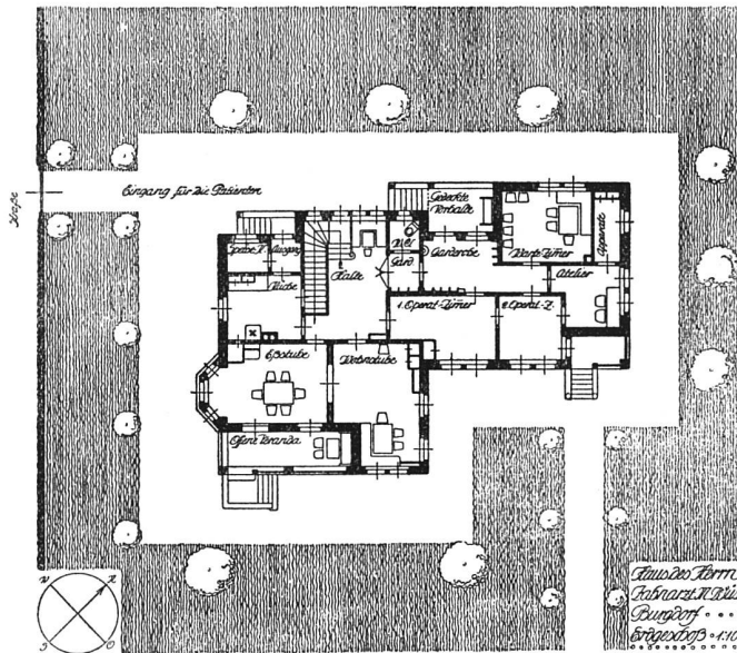
Architekt (B. S. U.) Hector Egger, Langenthal. — Erdgeschoßgrundriß. — Maßstab 1:400
