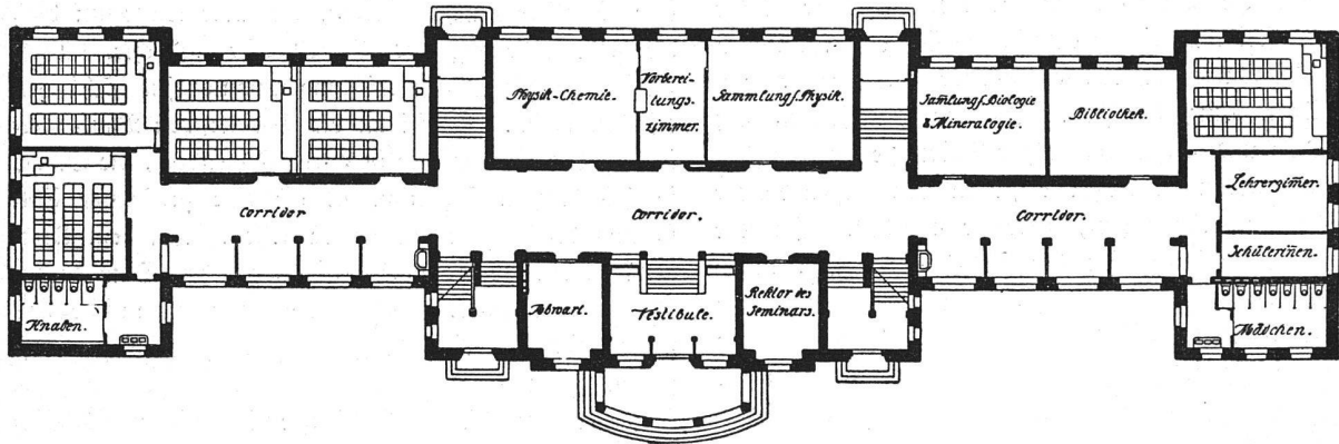
Grundrisse des Erdgeschosses, des ersten Obergeschosses und des Dachstodes. Maßstab 1:500 Das Selgki-Schulhaus in Aarau. Architekten Bracher, Widmer und Daxelhofer in Bern.
