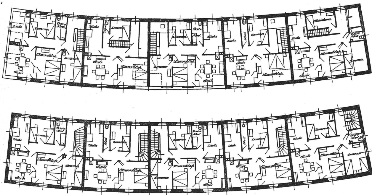
Fünfhäusergruppe. — Grundrisse der beiden Obergeschosse 1:300
