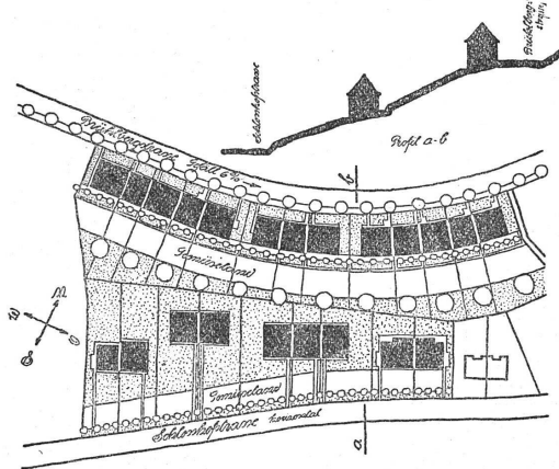
Zur Ueberbauung des Brühlbergareals in Winterthur - Architekten W. S. A. Fritsch & Jangerl in Winterthur Geometrische Ansicht - Ansichten und Querschnitt der Fünfhäusergruppe 1:200 - Lageplan und Querschnitt 1:2000
