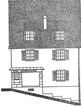
Zur Ueberbauung des Brühlbergareals in Winterthur - Architekten W. S. A. Fritsch & Jangerl in Winterthur Geometrische Ansicht - Ansichten und Querschnitt der Fünfhäusergruppe 1:200 - Lageplan und Querschnitt 1:2000
