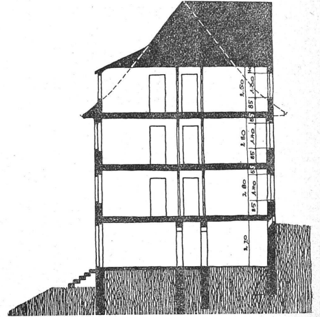
Zur Ueberbauung des Brühlbergareals in Winterthur - Architekten W. S. A. Fritsch & Jangerl in Winterthur Geometrische Ansicht - Ansichten und Querschnitt der Fünfhäusergruppe 1:200 - Lageplan und Querschnitt 1:2000
