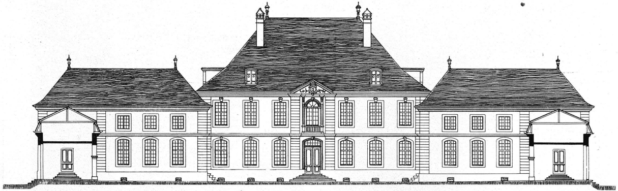
Schloss Hindelbank bei Bern. — Längsschnitt und Querschnitt durch den Hof. — Massstab 1:300. Aufgenommen von Schülern des kantonalen Technikums zu Burgdorf unter Leitung von A. W. Müller (Burgdorf), Winterthur.
