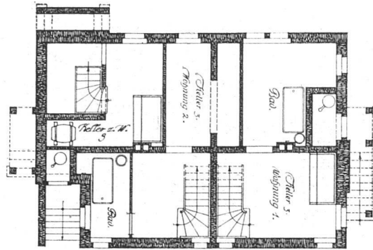
Kellergeschoss
