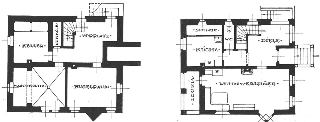
Kellergeschoss
