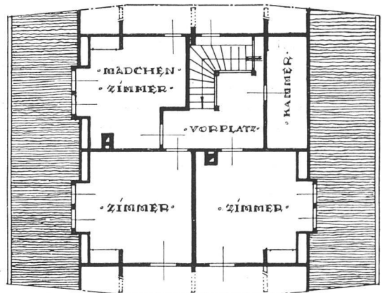
Dachstock
