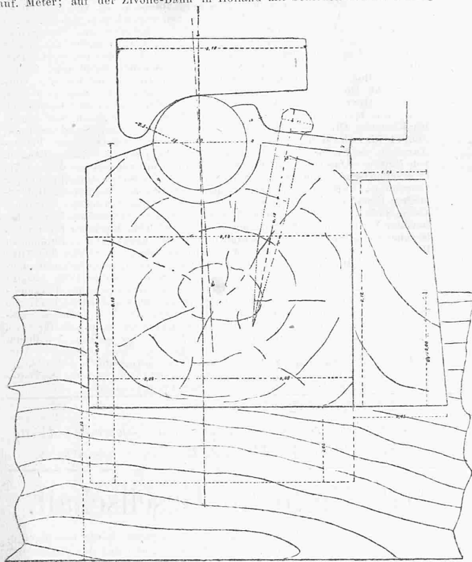
Durchschnitt durch die Mitte einer Längschwelle. Fig. 19.
