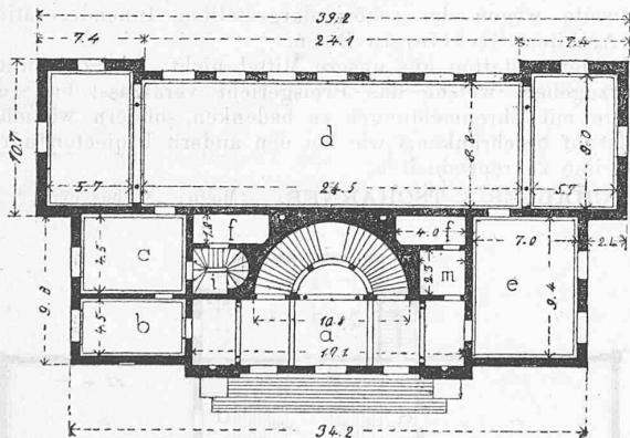
Erhöhtes Erdgeschoss. Maasstab 1 : 500.
