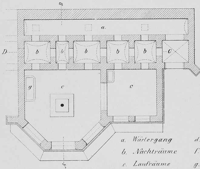
Grundriss
