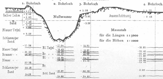
Querprofil in der Brückenaxe
