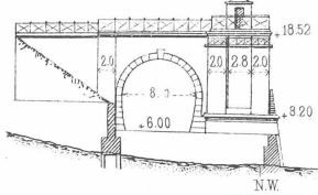
Querprofil in der Brückenaxe
