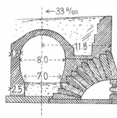
Project von Baudirector Hellwig in Wien Szegediner Widerlager Schnitt
