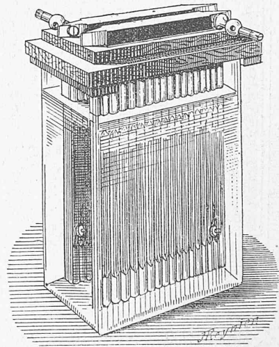
Fig. 2. Accumulateur plomb-plomb modèle de démonstration à une paire de plaques.
