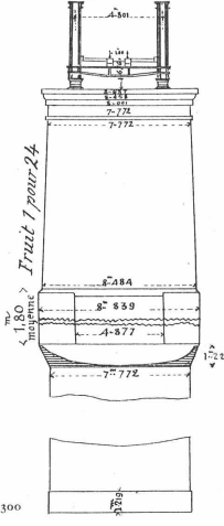
Fig. 2. Élévation transversale.
