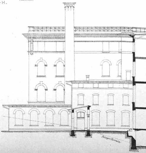
SCHNITT C-D
