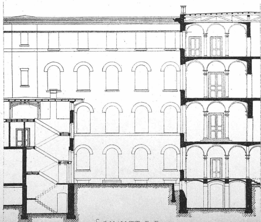
SCHNITT E-F.
