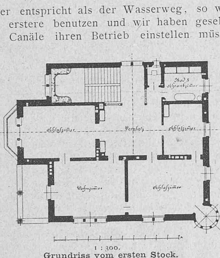
Grundriss vom ersten Stock.
