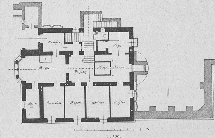
Grundriss vom Untergeschoss.
