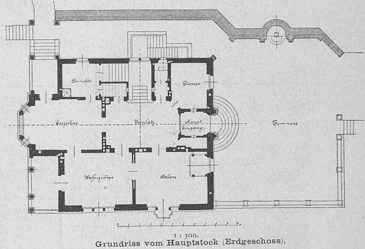
Grundriss vom Hauptstock (Erdgeschoss).
