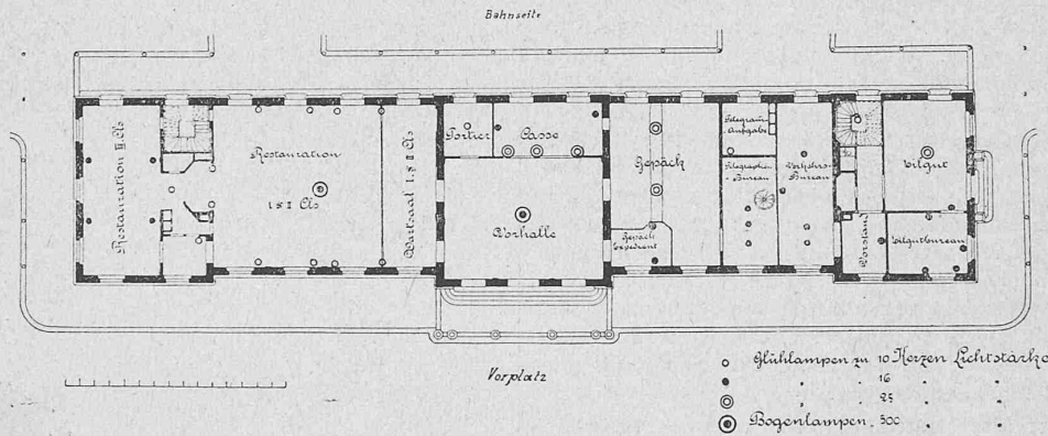
Grundriss vom Erdgeschoss. 1 : 500. — 2 mm = 1 m.
