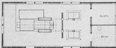
Fig. 6. Grundriss. 1 : 250. — 4 mm = 1 m.
