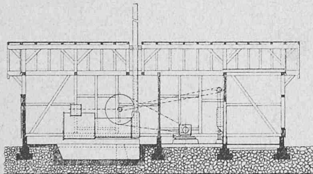
Fig. 5. Längenschnitt.
