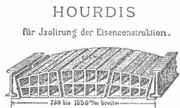
HOURLIS für Isolierung der Eisenkonstruktion.
