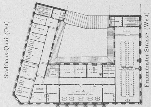
Kappeler-Gasse (Nord). Grundriss vom ersten Stock.
