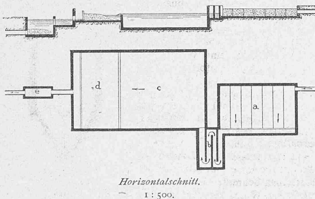
Fig. 13 und 14. Filtrationsanlage. System Petri. Vertikalschnitt.
