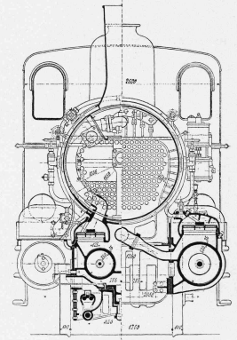
Mastab 1:40. Querschnitt der viercylindrigen Verbund-Schnellzugs-Lokomotive A 3 T Nr. 202 der Gotthardbahn.
