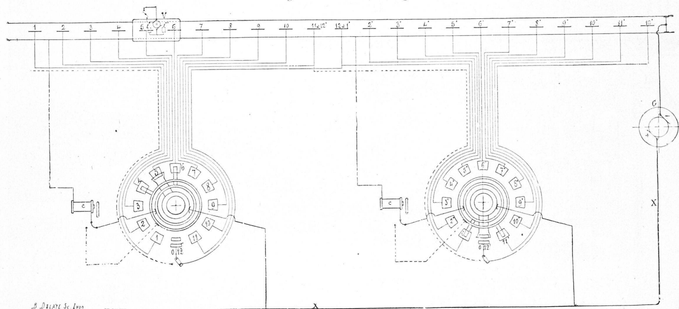
Fig. 1. Strom-Verteilung.
