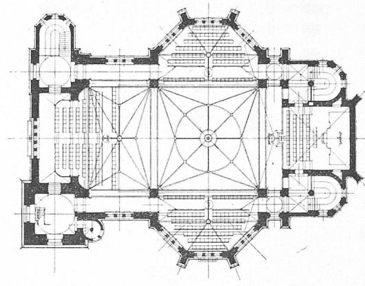
Emporen-Grundriss.
