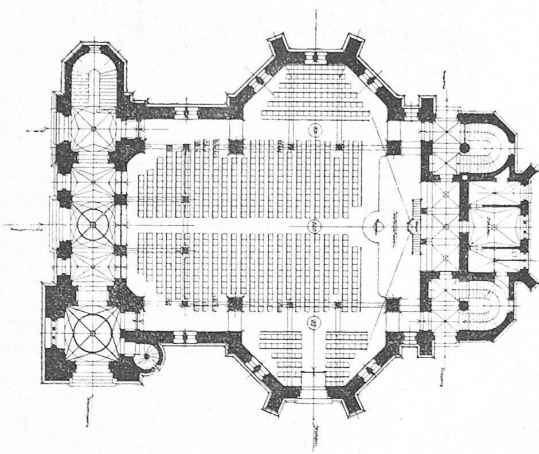
Erdgeschoss-Grundriss.
