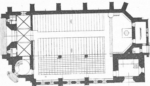
Erdgeschoss-Grundriss. Masstab 1 : 600.
