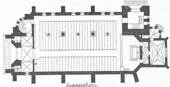
Erdgeschoss. Masstab 1 : 666 \frac{2}{3} .
