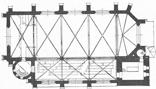
Emporen-Grundriss.
