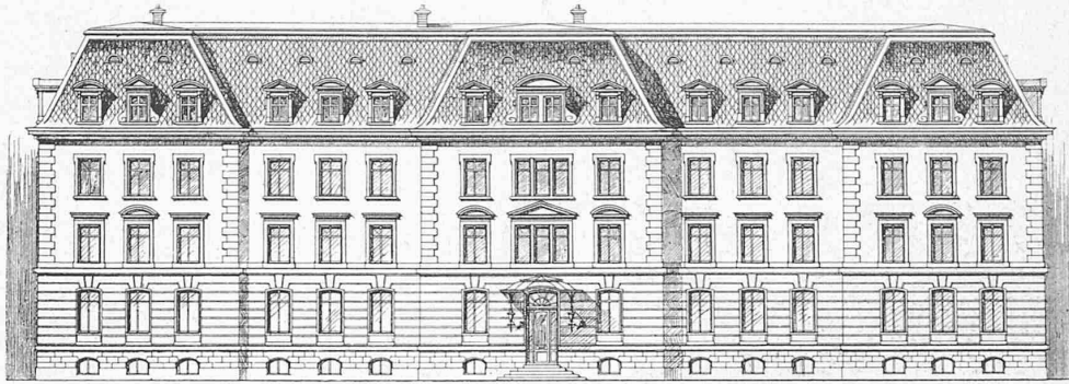
Ost-(Haupt)-Fassade.
