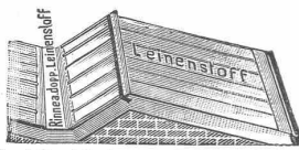
Shed-Dachdeckung mit Rinnenbekleidung
