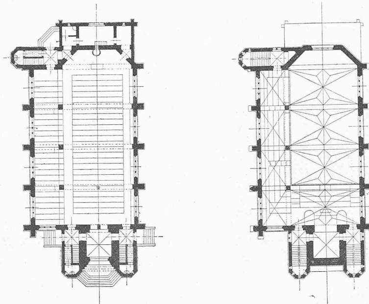
Erdgeschoss Grundriss.
