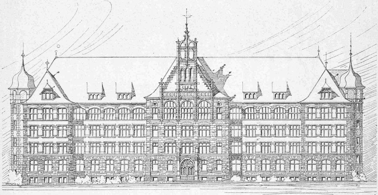
Hauptfassade 1 : 500.
