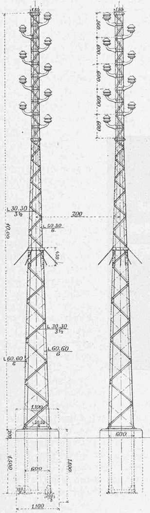
Fig. 19a. Masten der Hochspannungsleitung 1:80.
