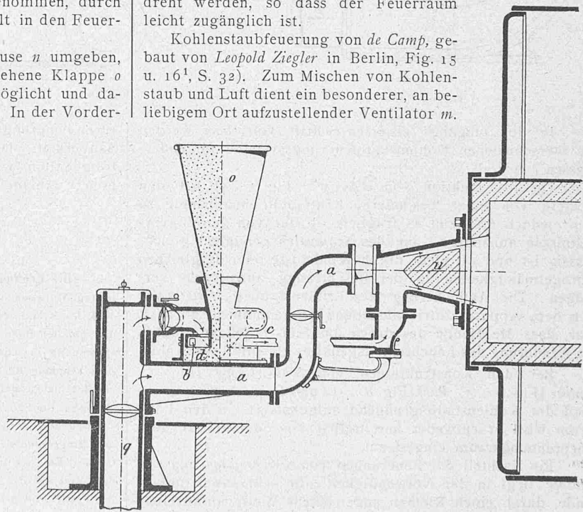
Fig. 13 u. 14. System Friedeberg.
