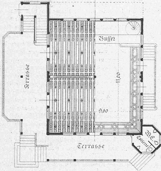
Plan du rez-de-chaussée. 1 : 200.
