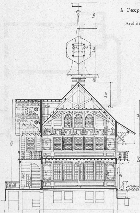
Coupe.
