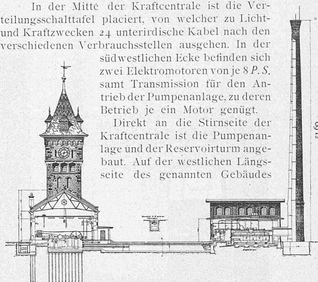
Fig. 37. Kraftzentrale und Dampfkesselhaus. — Verbindungskanal. Masstab 1:800.
