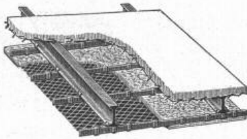
Deckenkonstruktion Hurdslatten und Gipsplatten.
