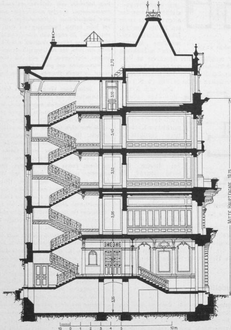
Querschnitt 1: 500.
