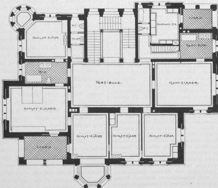
Grundriss vom I. Stock. 1:250.
