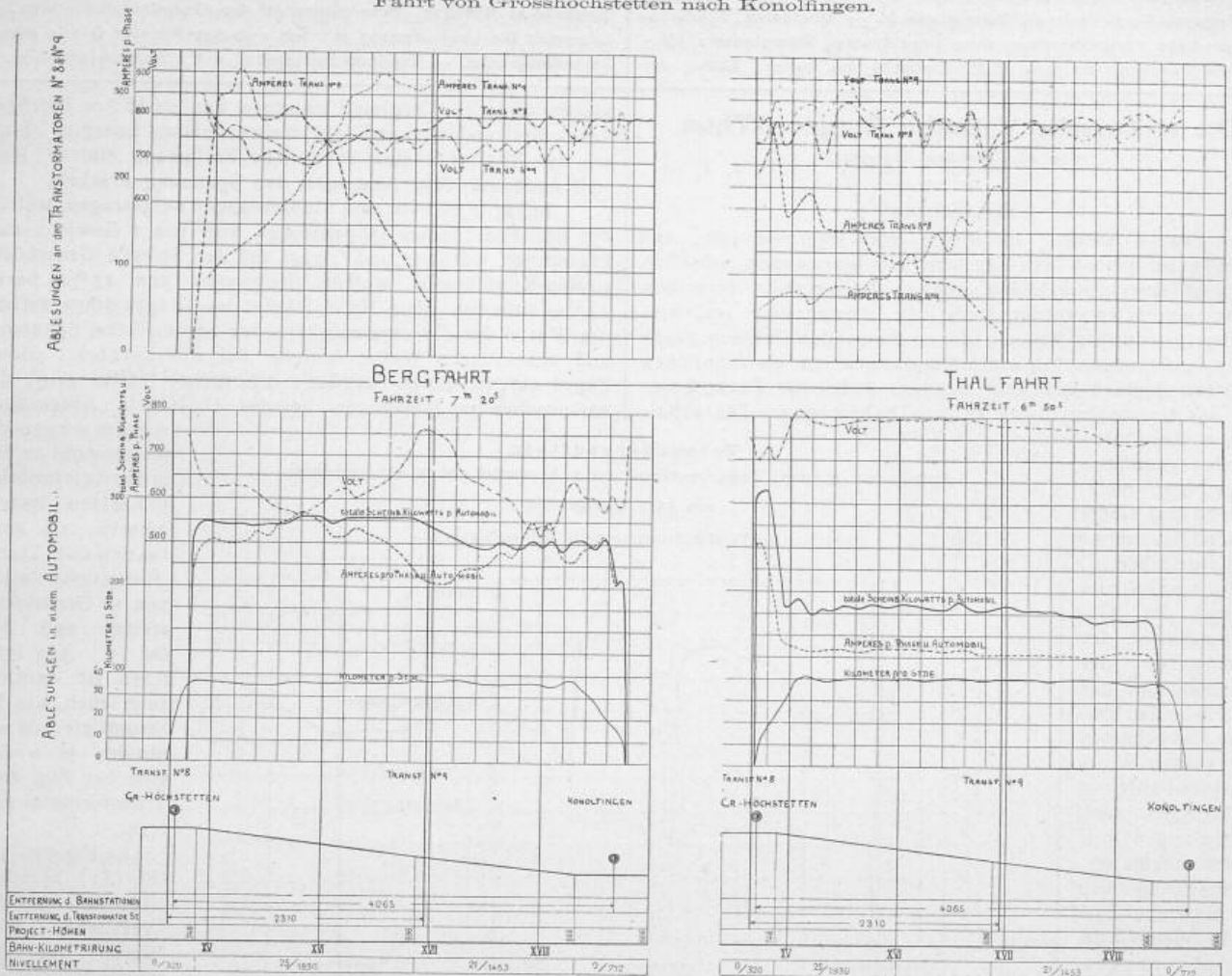
Fig. 2. Kurven der Stromstärke, Spannung, Geschwindigkeit und scheinbaren kwh .
