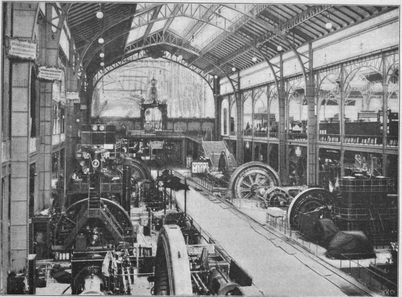
Fig. 7. Maschinensaal der Kraftcentrale «La Bourdonnais» (Franz. Sektion).
