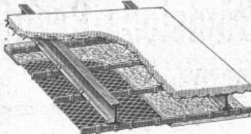
Deckenkonstruktion Hardis und Gipsplatten.
