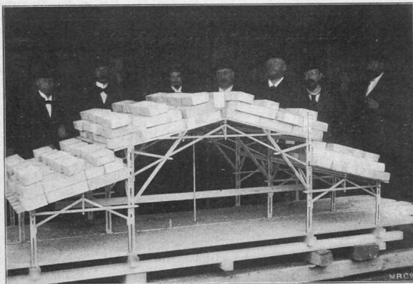
Modell 1:20 für die Festhalle des eidg. Schützenfestes 1901 in Luzern. (Nach dem Entwurf von Ing. Lubini in Luzern.)
