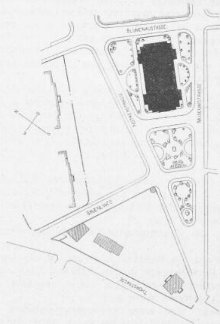
Lageplan 1 : 2500.
