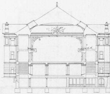
Querschnitt 1:500.
