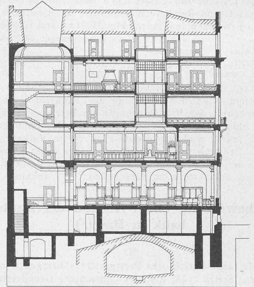
Längsschnitt. 1 : 400.
