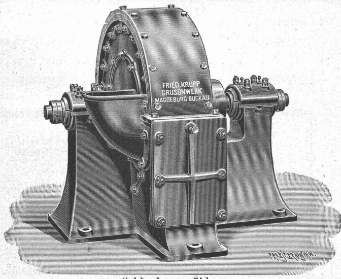
Schlagkreuzmühle.
