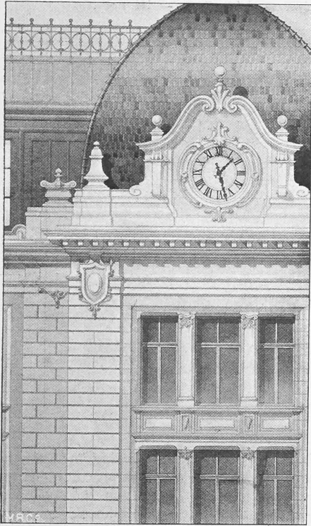
Entwurf von Arch. Ernst Hünervadel in Bern. Fassaden-Detail. — 1 : 50.
