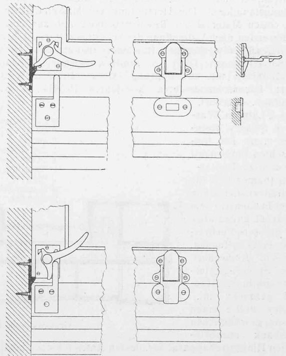
Fig. 3. Feststell-Hebel und Kuppelungsvorrichtung der Wagenfenster.
