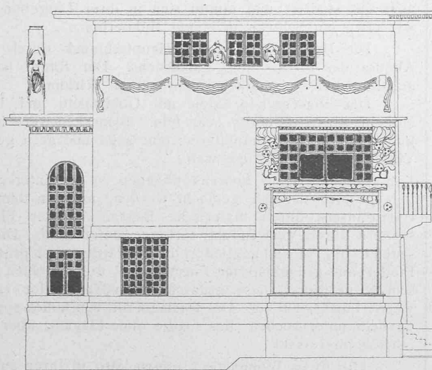
Abb. 15. Haus Habich. — Nordfront. — 1 : 150. Architekt: Prof. Olbrich.
