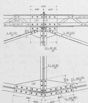
Fig. 17. 1 : 50.
