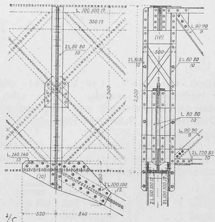
Fig. 15. Masstab 1 : 50.
