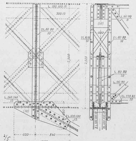
Fig. 15. Masstab 1 : 50.
