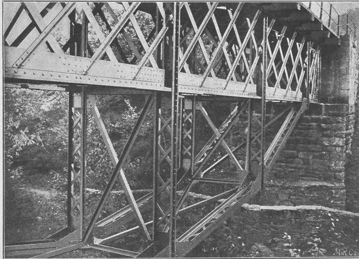
Fig. 11. Verstärkte Galli-Brücke.
